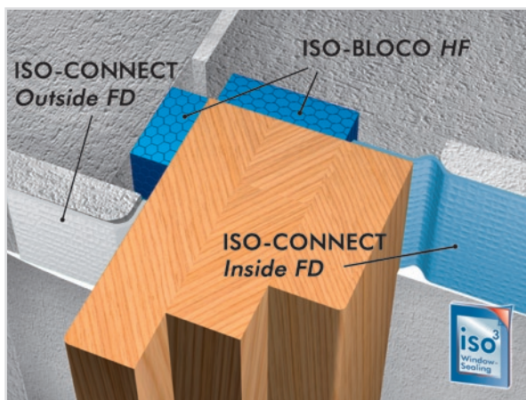
Exemplu de instalare iso 3 -Sistem etansare a ferestrei
